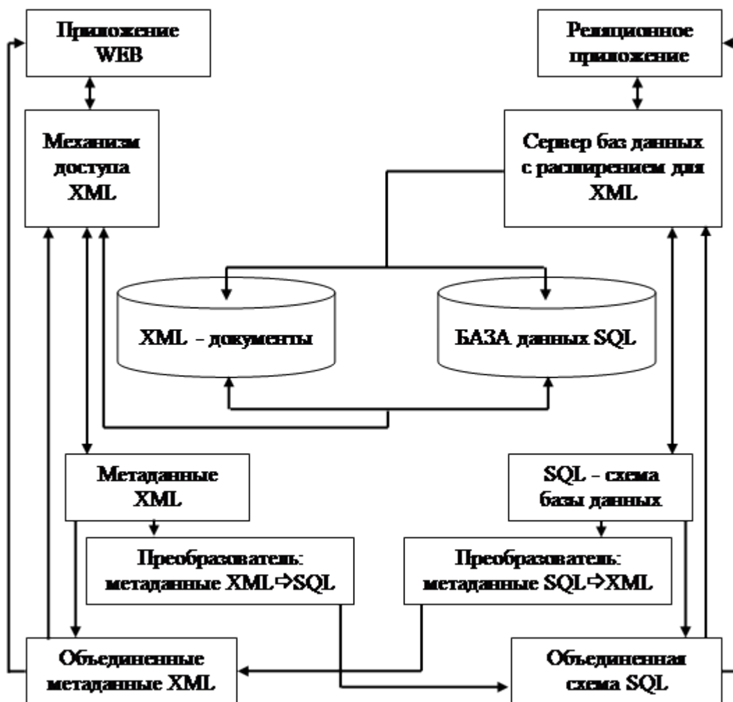
Рис. 1. Упрощенная архитектура системы, обеспечивающей интеграцию информационных ресурсов XML и SQL
